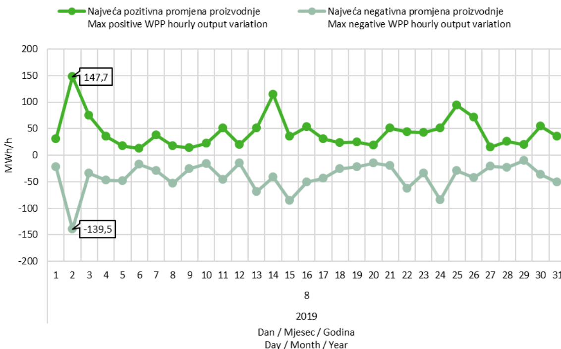
Slika 9 Maksimalna pozitivna i maksimalna negativna promjena satne proizvodnje VE u kolovozu 2019. godine
