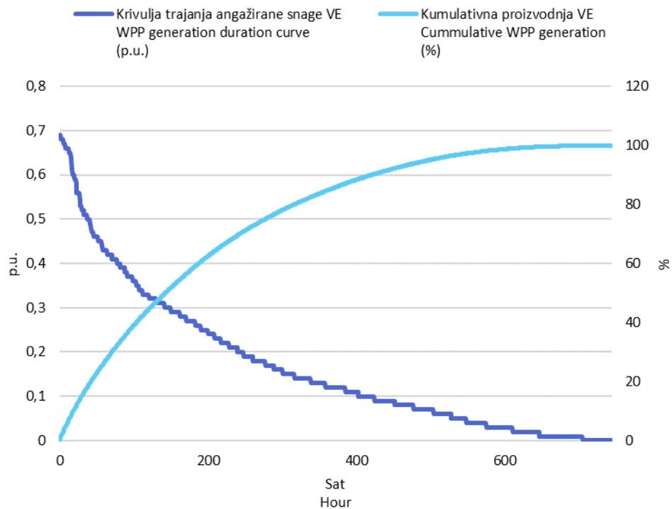
Slika 3 Krivulja trajanja angažirane snage svih VE i kumulativna proizvodnja VE u kolovozu 2019. godine u jediničnim vrijednostima
