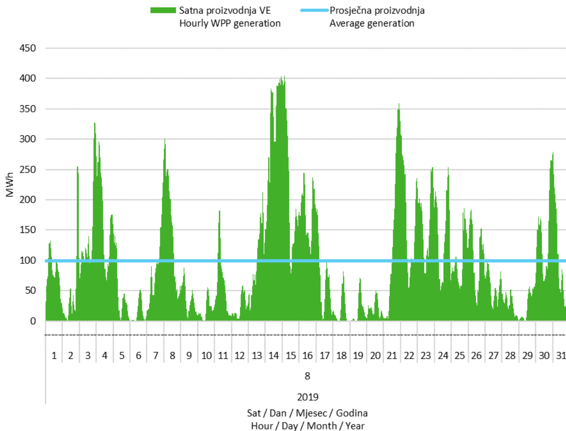
Slika 2 Satna proizvodnja svih vjetroelektrana u kolovozu 2019. godine
