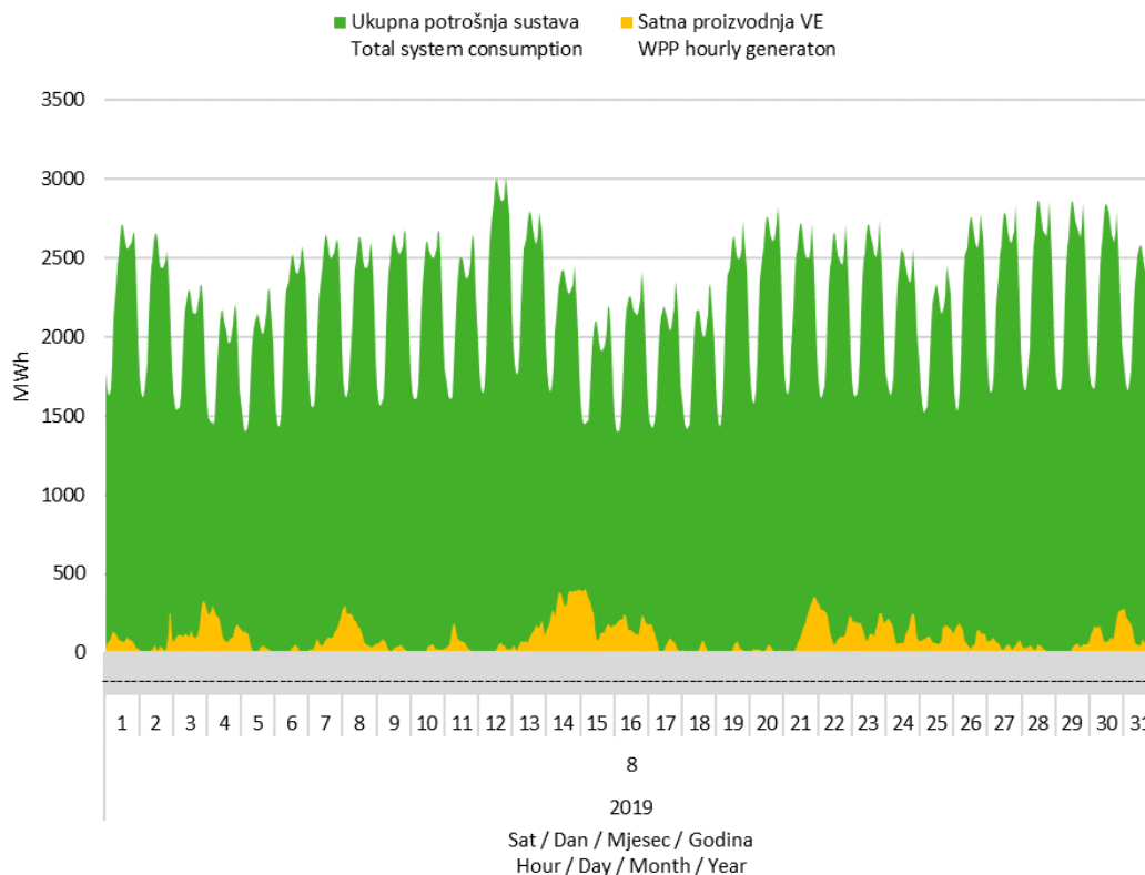
Slika 7 Usporedba satnog dijagrama opterećenja sustava i proizvodnje vjetroelektrana u kolovozu 2019. godine
