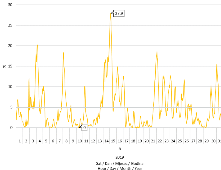
Slika 8 Udio proizvodnje vjetroelektrana u pokrivanju satnog opterećenja elektroenergetskog sustava u kolovozu 2019. godine
