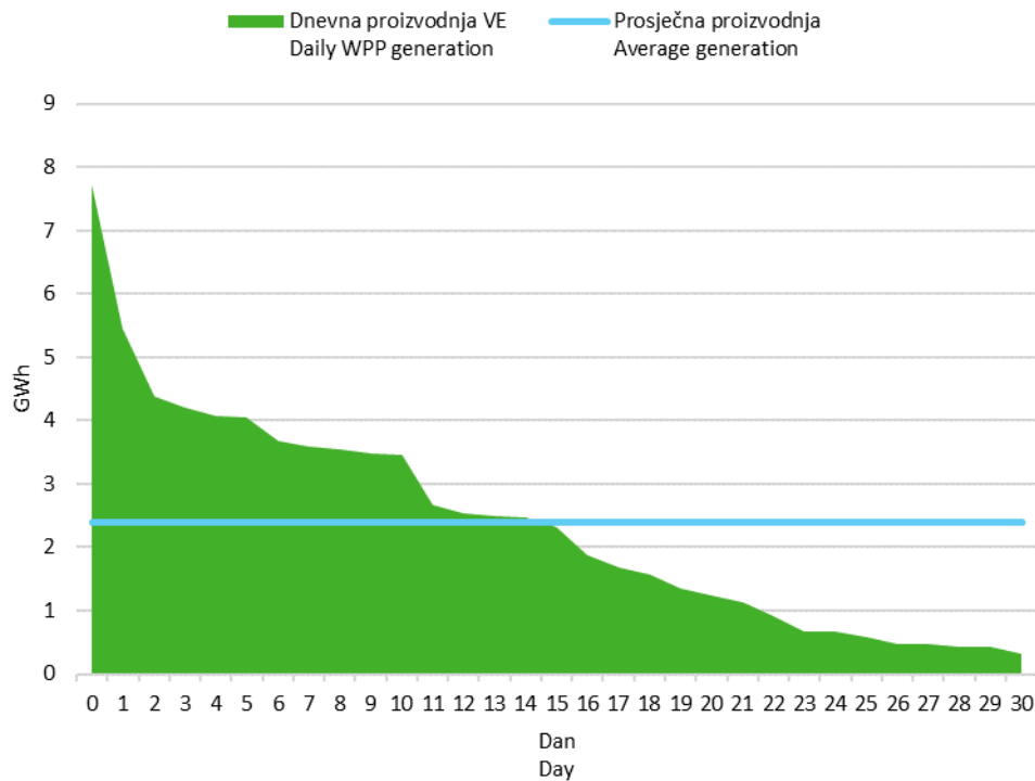
Slika 6 Krivulja trajanja dnevne proizvodnje vjetroelektrana u kolovozu 2019. godine
