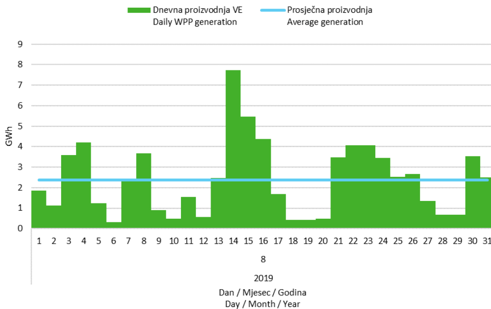
Slika 5 Dnevna proizvodnja svih vjetroelektrana u kolovozu 2019. godine
