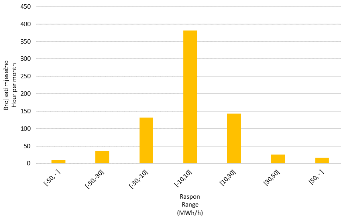
Slika 10 Statistička raspodjela satnih promjena proizvodnje VE u kolovozu 2019. godine
